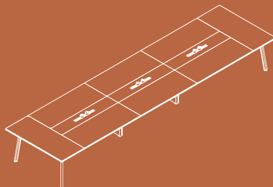
YCT-04 4800*1500*750 5700*1500*750 6600*1500*750
