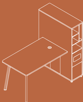
YCT-05 1900*900*900/1700 2400*900*900/1700
