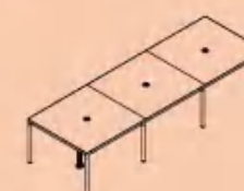
CHCT-04 3600*1200*750 4200*1200*750
