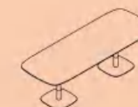
CHCT-02 1800*900/1000*720 2000*900/1000*720 2200*900/1000*720 2400*900/1000*720
