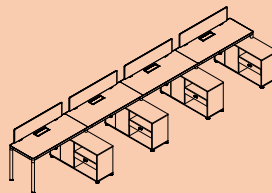
C-CHST-D-04 4800*1200*750 5600*1200*750
