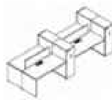
C-ANST-S-02 3600*1400*750/1200 3800*1400*750/1200
