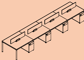
A-CHST-S-04 4800*1200*750 5600*1200*750
