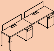
A-CHST-D-02 2400*(600/700)*750 2800*(600/700)*750
