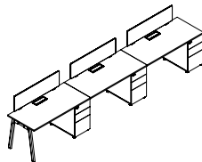
A-BST-D-03 3600W*700D*750H 4200W*700D*750H
