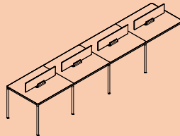
B-CHST-S-05 4800*1200*1050 5600*1200*1050
