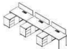
C-RIST-03 4200W*600D*750H 4200W*700D*750H 4500W*700D*750H
