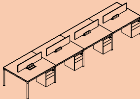
B-CHST-S-04 4800*1200*750 5600*1200*750
